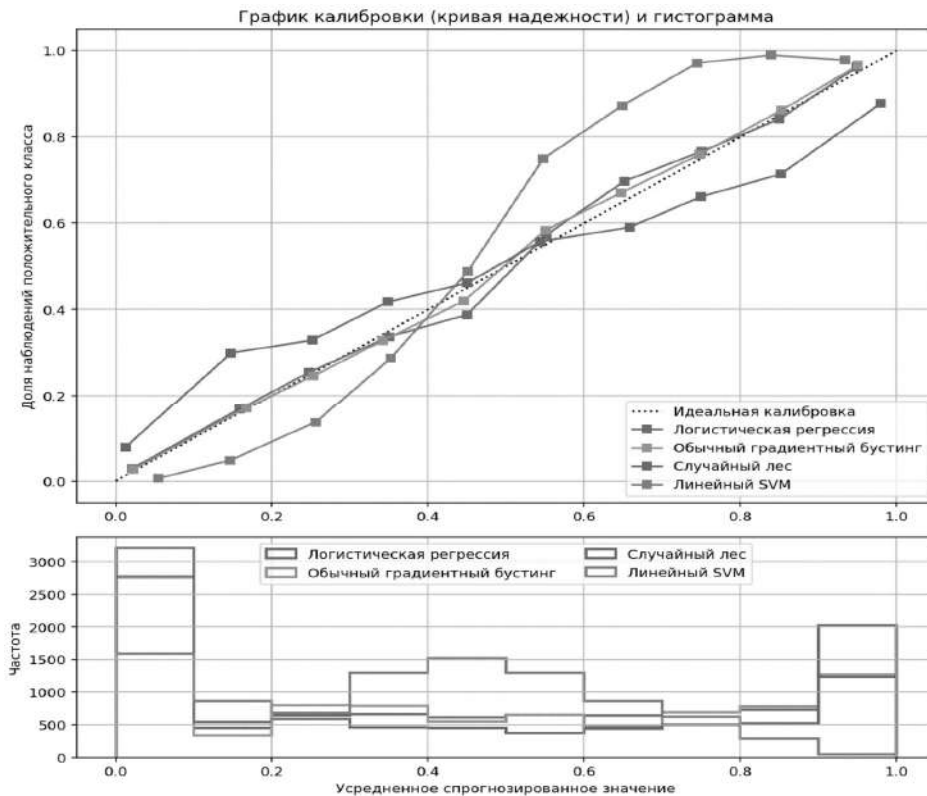
Пример сравнения качества калибровки вероятности положительного класса для трех различных классификаторов: логистической регрессии, градиентного бустинга и случайного леса (адаптация scikit-learn.org).
